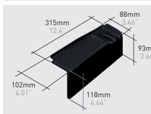
Q99*K | Dachówka krawędziowa prawa Visum3
