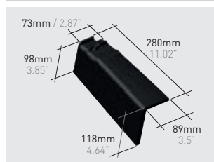
Q101*K | Dachówka krawędziowa lewa Visum3
