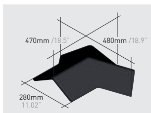
Q111*K | Trójkąt poddaszowy 120° kalenicy
