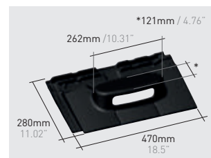
Q97*K | Dachówka przelotowa kominowa/sanitarna Visum3
